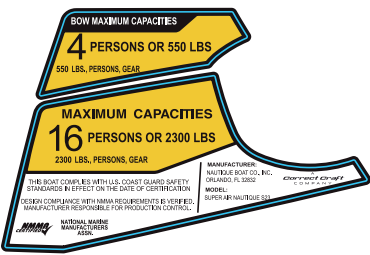
S23 P/N 220673
